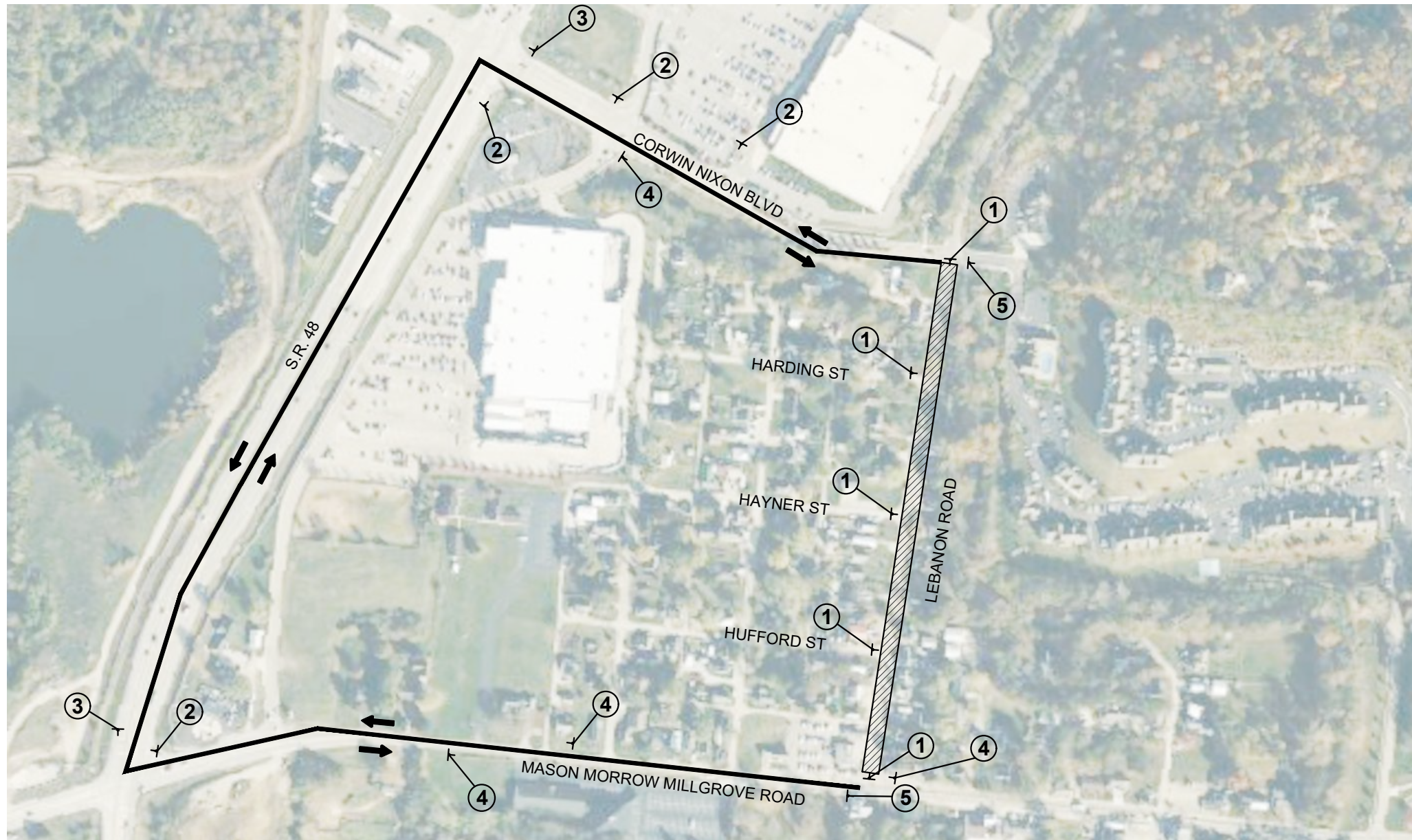
DETOUR PLAN
